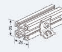
Монтажный профиль 48630 серебристый
