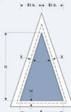
PL 32 Треугольник PLE 32 Треугольник
