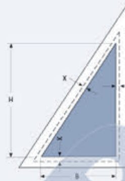
PL 33 Треугольник (1 скос) PLE 33 Треугольник (1 скос)
